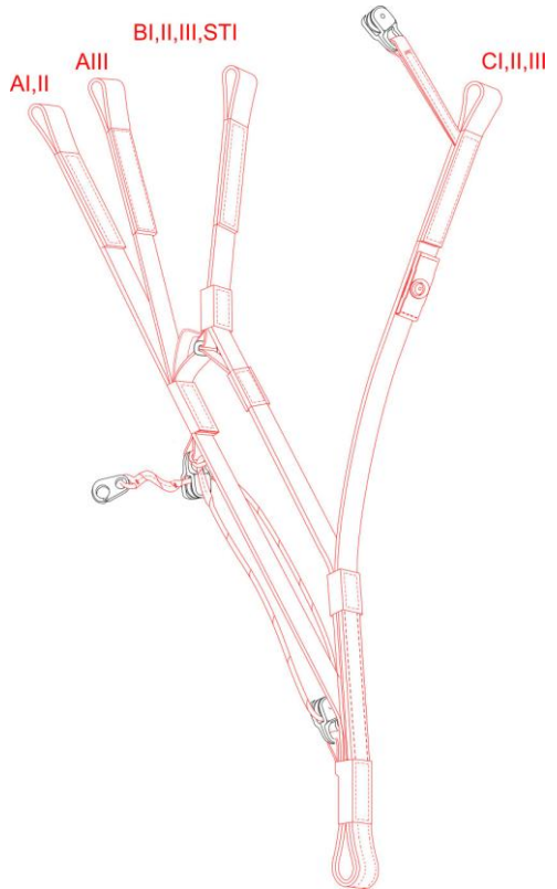
Abbildung 2: Tragegurte des UP Ascent 3
